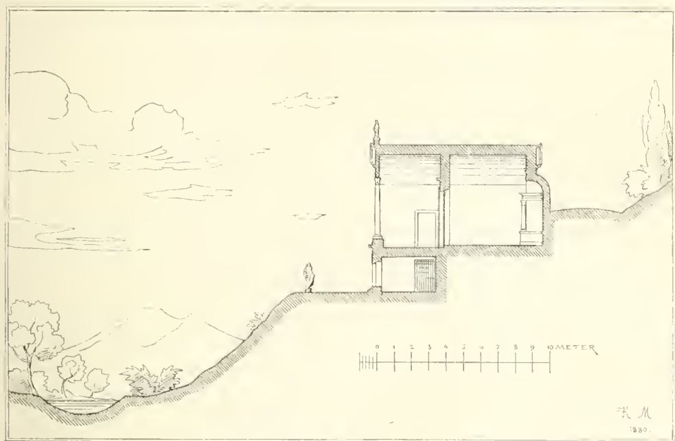
Fig. 2. Der Clitumnustempel bei Trevi. Durchschnitt.
